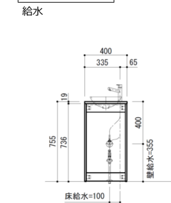
断面図 (正面)
